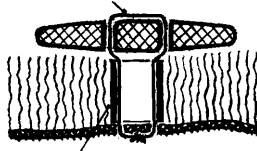
ПЛАСТМАССОВАЯ ТРУБКА
