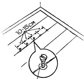
ОТВЕРСТИЕ РАЗЗЕНКОВАТЬ
